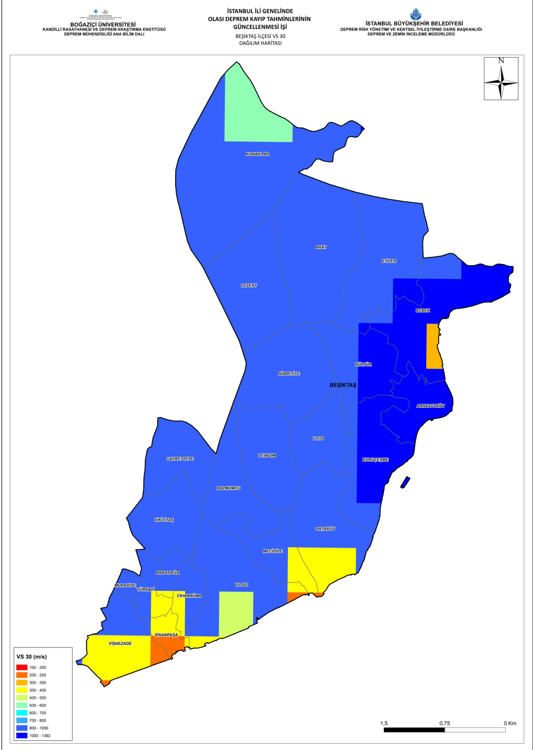
Şekil 4-1: Beşiktaş İlçesi VS 30 Dağılımı
