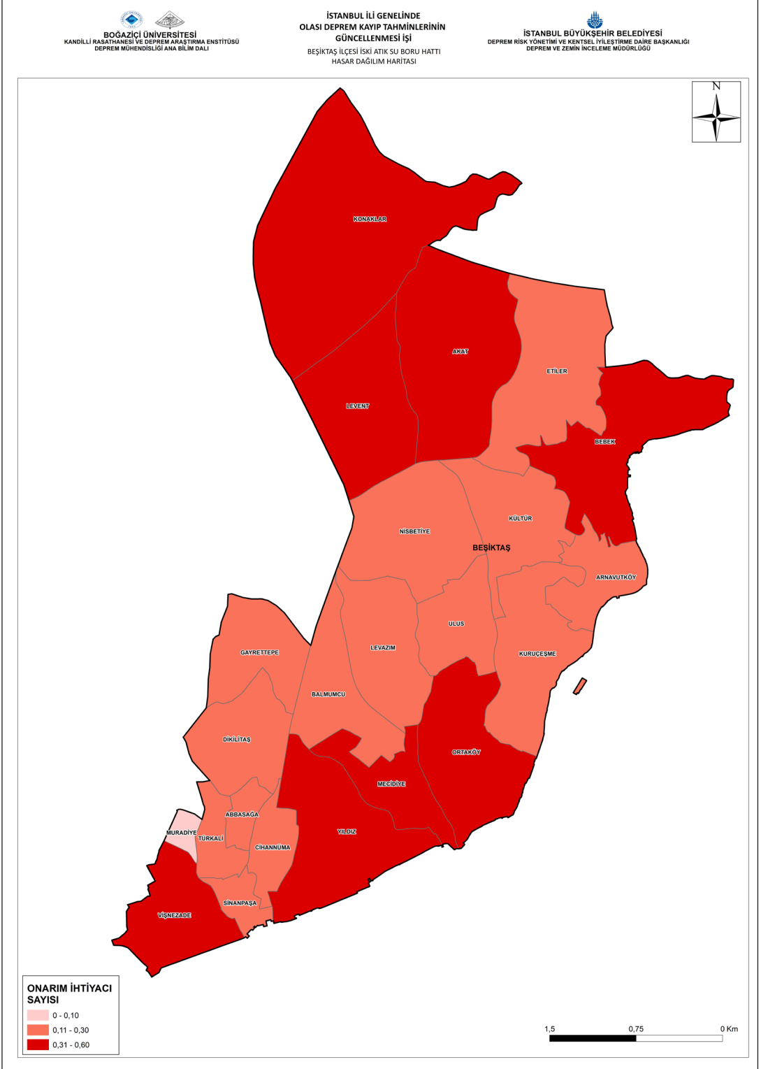
Şekil 5-11: Mw=7.5 Senaryo Depremi İçin Beşiktaş İlçesi İSKİ Atık Su Boru Hatları Tahmini Onarım İhtiyacı Dağılım Haritası
