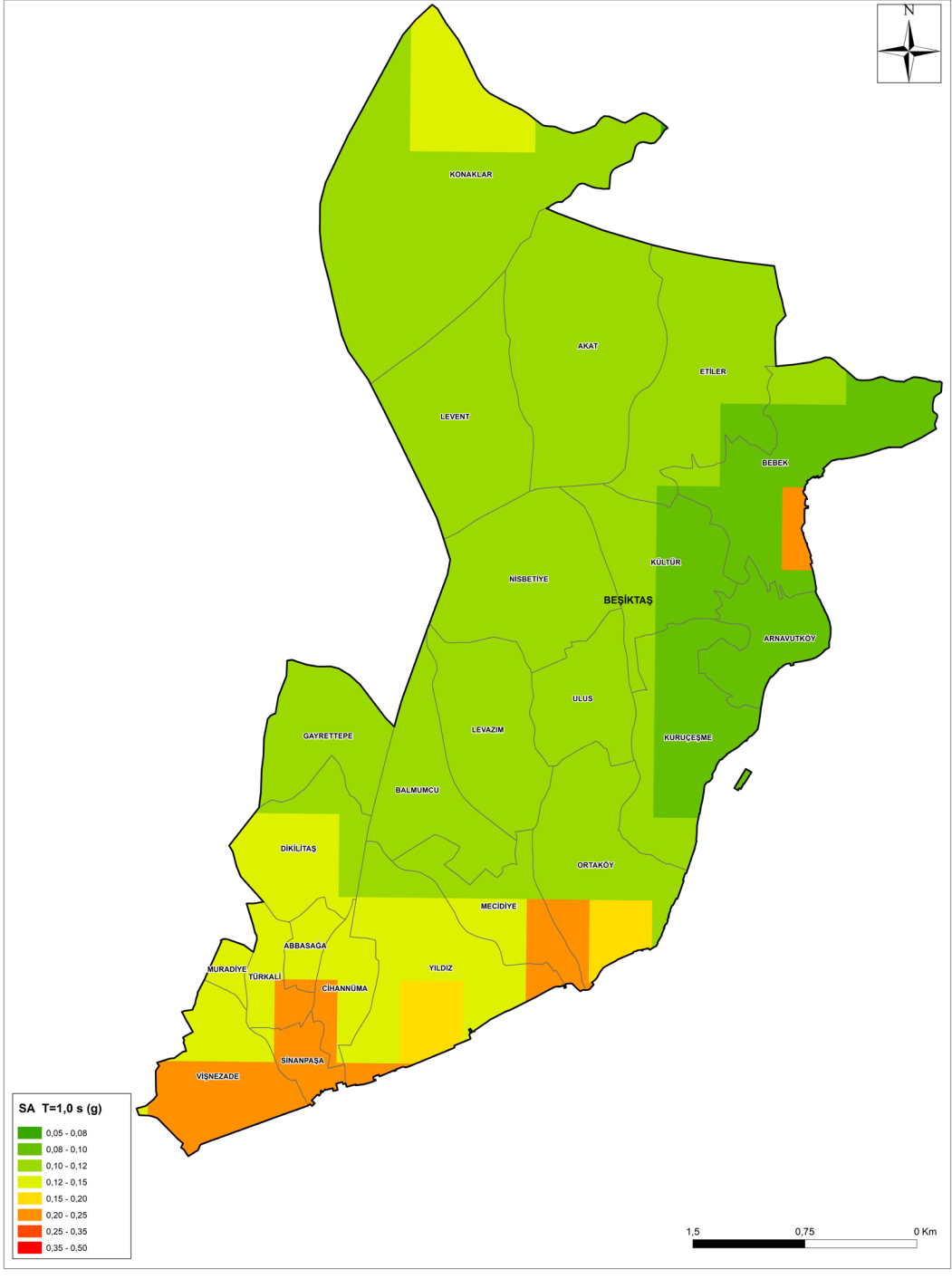
Şekil 4-7: Senaryo Depremi için Elde Edilen Beşiktaş İlçesi Zemin Bağımlı T=1,0 s için Spektral İvme Dağılımı
