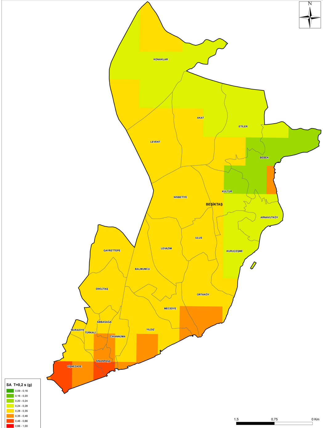
Şekil 4-6: Senaryo Depremi için Elde Edilen Beşiktaş İlçesi Zemin Bağımlı T=0,2 s için Spektral İvme Dağılımı
