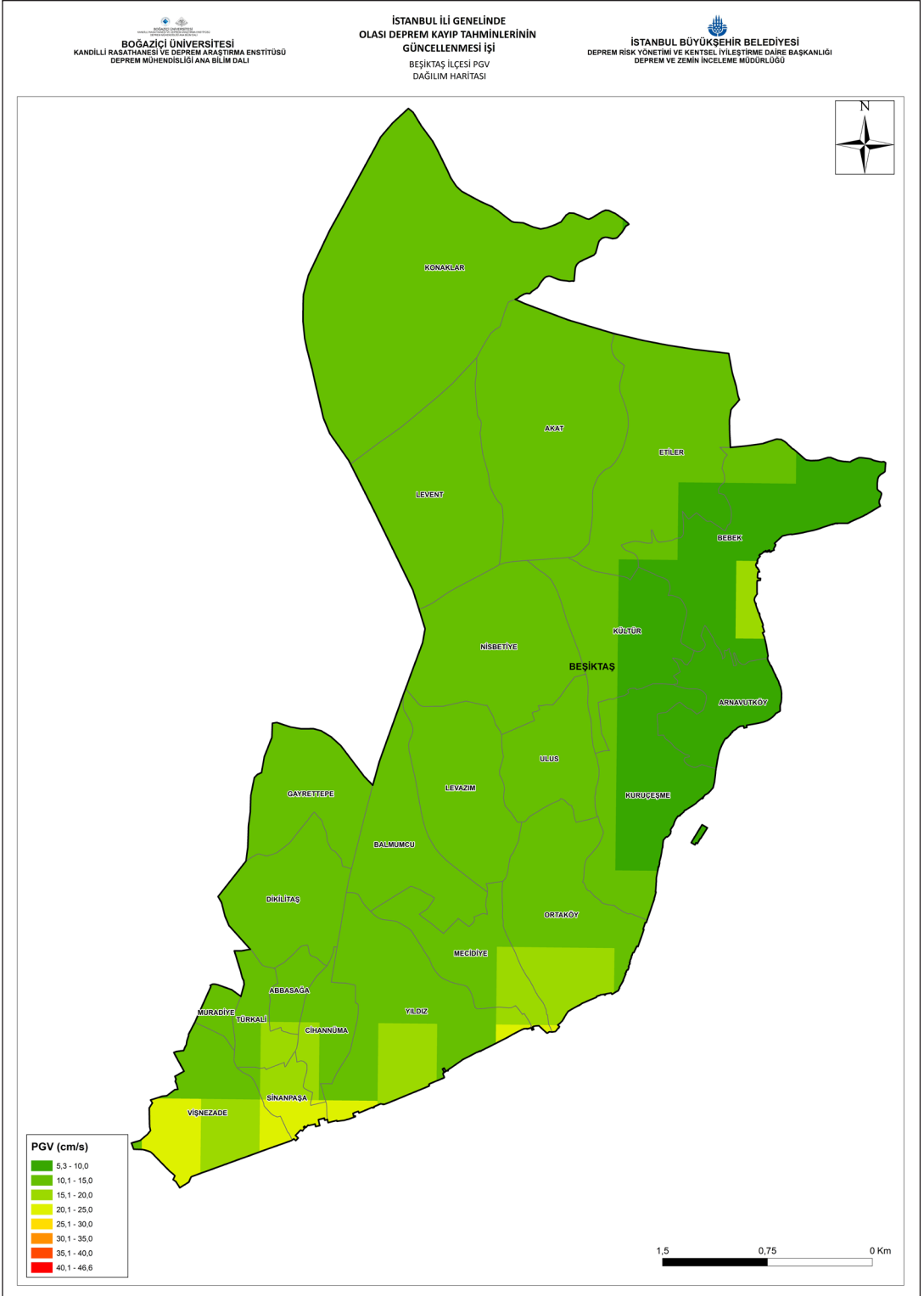
Şekil 4-5: Senaryo Depremi İçin Elde Edilen Beşiktaş İlçesi Zemin Bağımlı Medyan En Büyük Yer Hızı (PGV) Dağılımı
